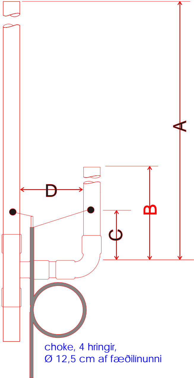
Mynd 1: J-póll úr hörðum 12mm eirrörum. Sjá töflu um mál. Ath. hlutföll í myndinni eru ekki rétt.
