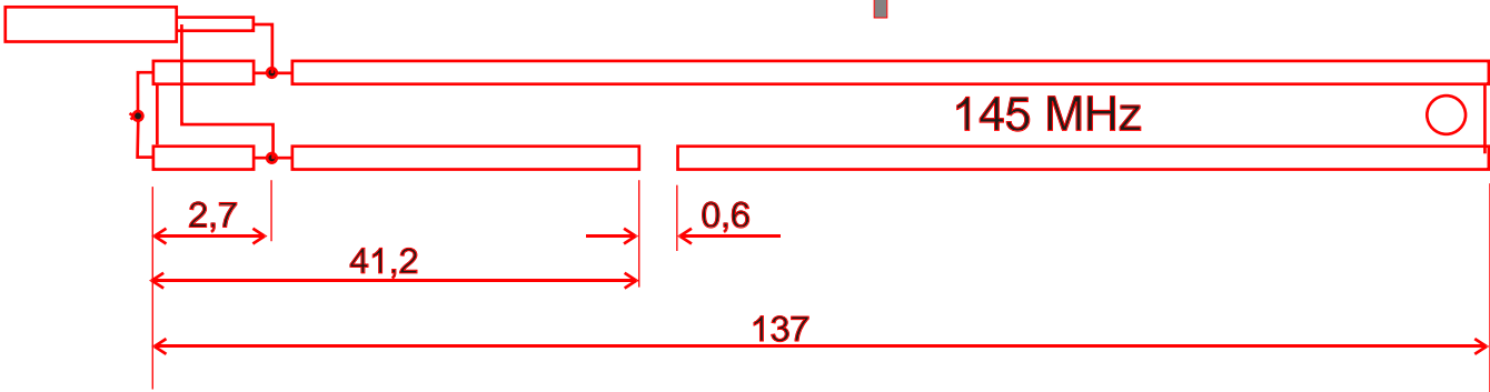
Mynd 2: J-póll úr 300 ohm tvíleiðara, allar lengdir eru í sm. Ath. hlutföll í myndinni eru ekki rétt.
